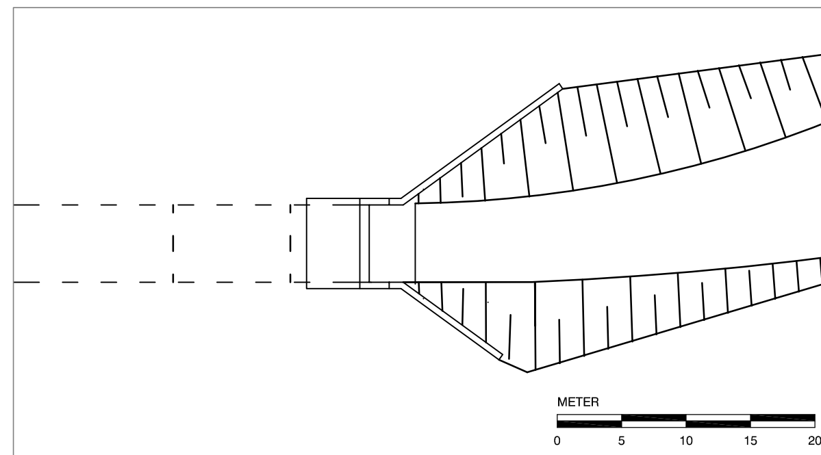
PLAN UTLØP
