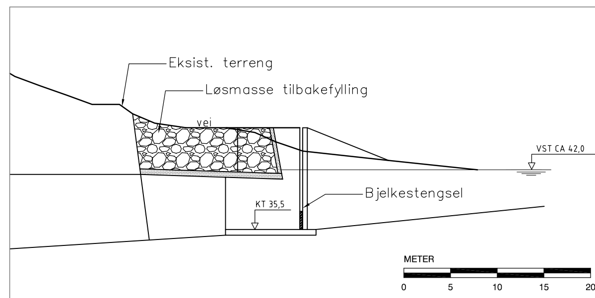
SNITT UTLØP
