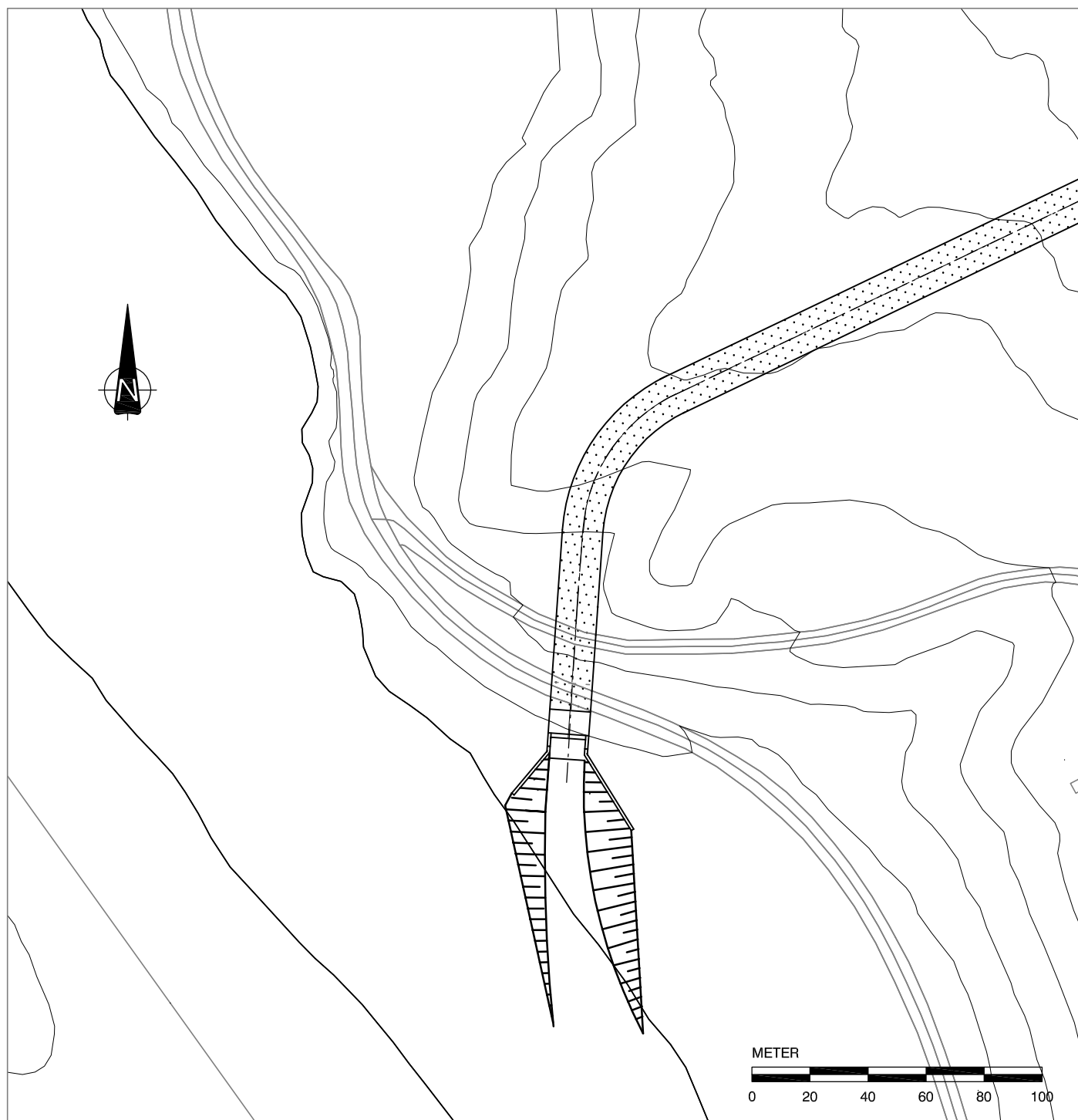
PLAN UTLØPSOMRÅDE
