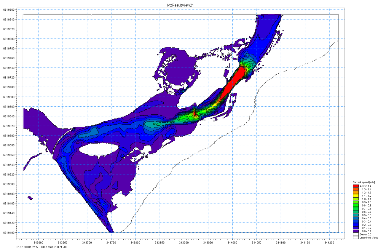
Figur 6-5. Vannføring 15 m 3 /s og minstevannføring 4 m 3 /s. Hastighet (m/s). (Multiconsult, 2013).
