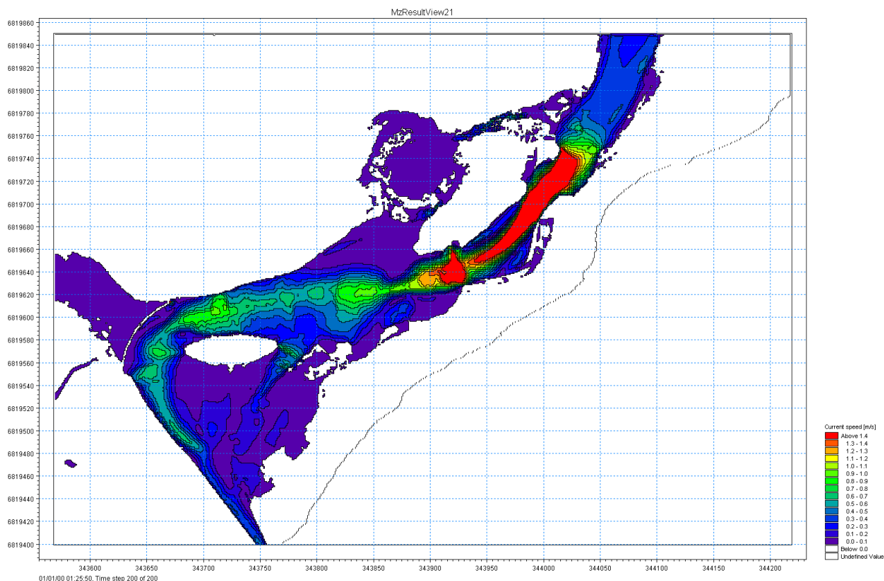
Figur 6-3. Vannføring 30 m 3 /s og minstevannføring 4 m 3 /s. Hastighet (m/s). (Multiconsult, 2013).
