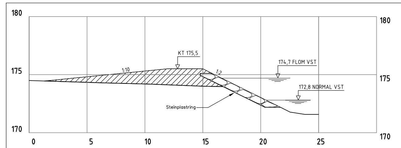
SNITT B-B
