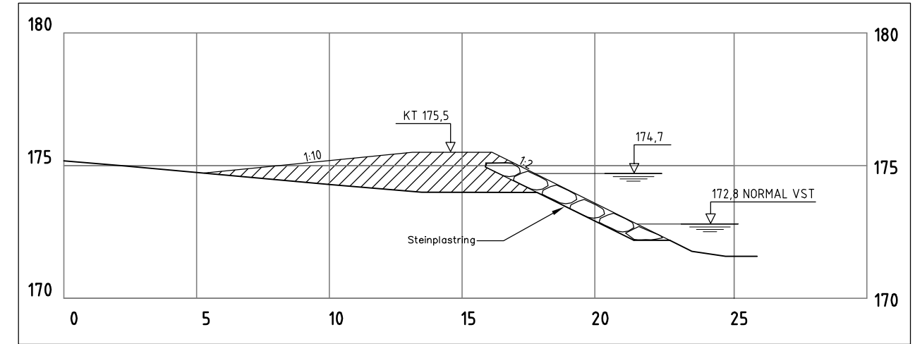
SNITT A-A
